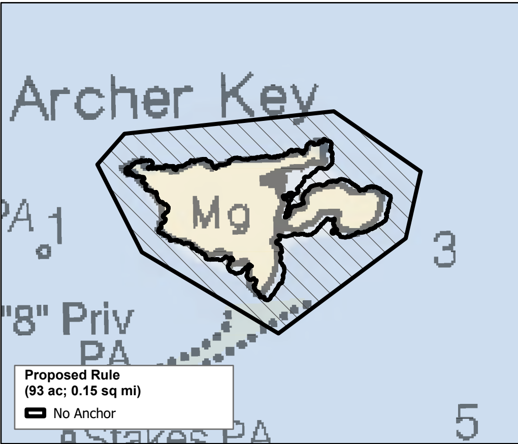
Marquesas Region
