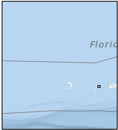
Marquesas Region
